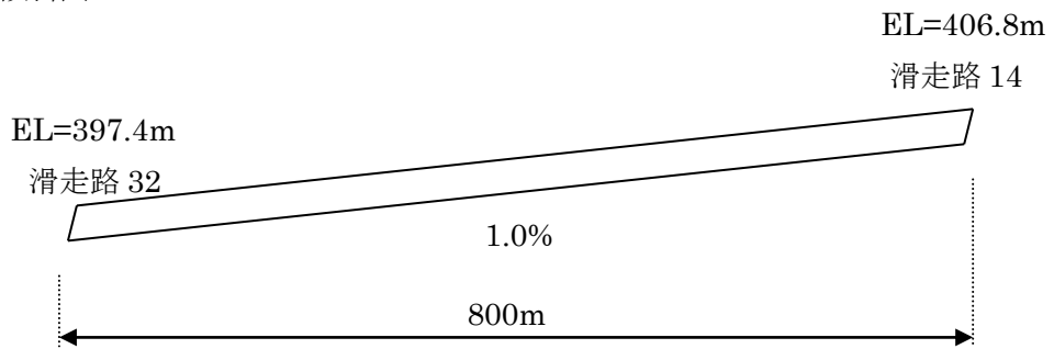
滑走路傾斜図
