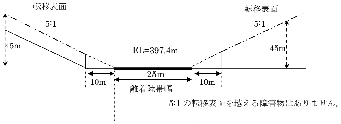
滑走路傾斜図
